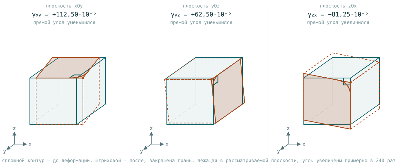
Рис. 1.5 — относительные угловые деформации: три элемента, на каждом показан сдвиг в своей координатной плоскости. Закрашена грань, лежащая в этой плоскости; у ближней вершины отмечены исходный прямой угол и угол после деформации. Сплошной контур — до деформации, штриховой — после; углы увеличены примерно в 240 раз (масштаб условный).
